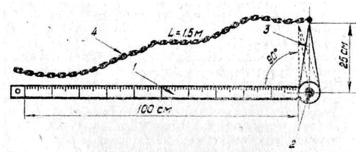
Рис. 2. Ледомер
