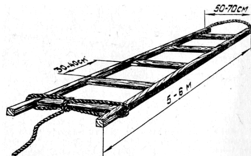
Рис. 9. Спасательная лестница № 1
